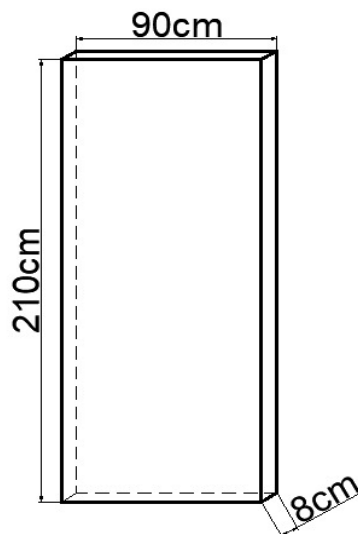
○ DETALHE DA PLACA DE CONCRETO
